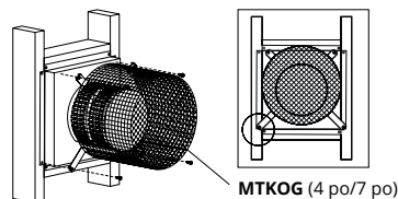
Figure 7.f Installation d'une grille thermique sur un chapeau MTO.
