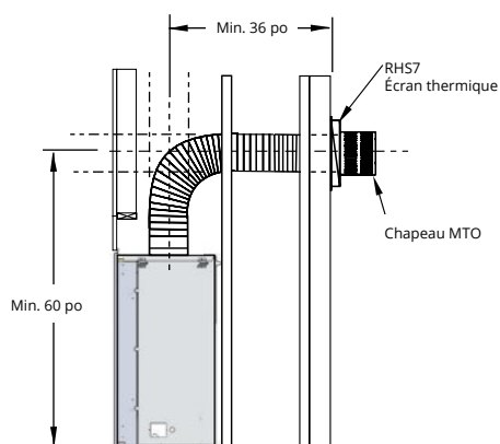
Figure 15.b Installation de l'écran thermique RHS7. (Exigences minimales)
