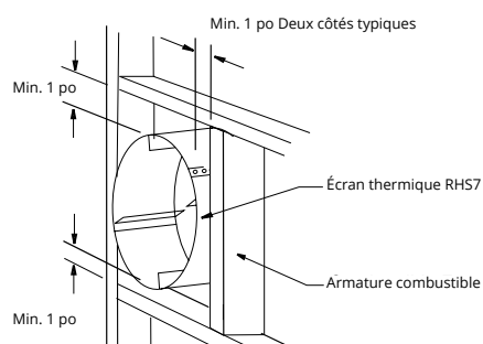
Figure 15.a Installation de l'écran thermique RHS7. (Installez-le en le glissant sur le tuyau de ventilation à l'endroit où il passe à travers la construction combustible).
