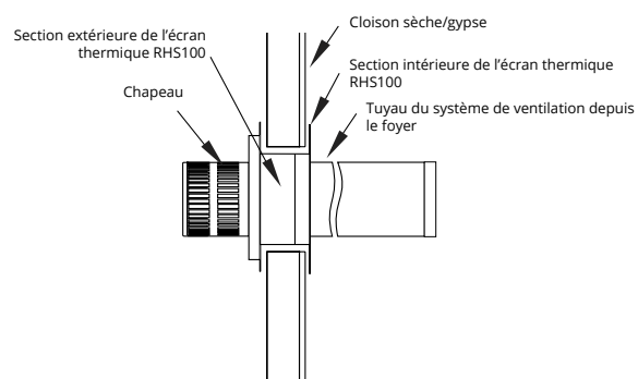
Figure 15.d Écran thermique. après avoir glissé la section extérieure en place.
