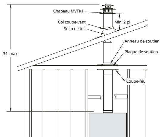
Figure 6. Évent supérieur, chapeau monté sur le toit sans déviation dans le parcours de ventilation.
