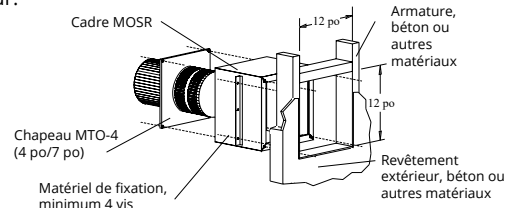
Figure 7.d Installation d'un chapeau MTO avec un cadre MOSR.
