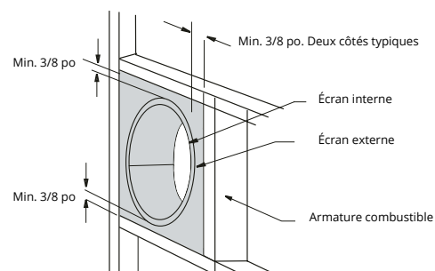
Figure 15.e Installation de l'écran thermique RHS100
