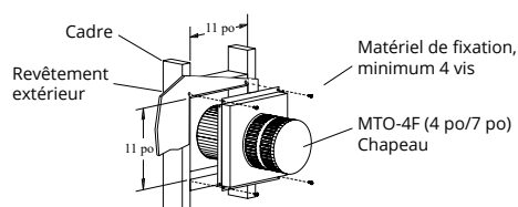
Figure 7. Installation d'un chapeau MTO4-F.
