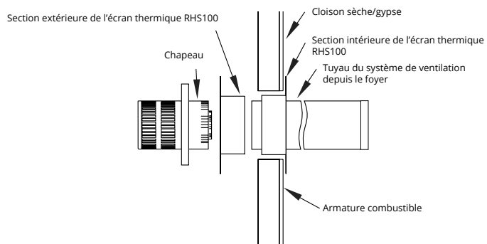
Figure 15.c Installation de l'écran thermique RHS100. (Installez-le en glissant la section extérieure sur le tuyau de ventilation à l'endroit où il passe à travers la construction combustible).
