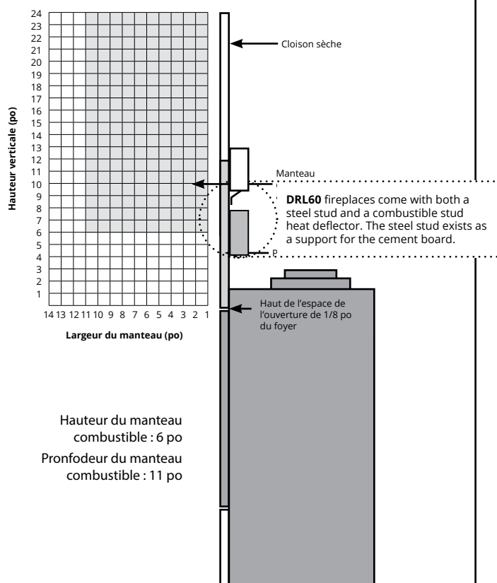
Figure 19. Manteaux combustibles et revêtements. (N'est pas à l'échelle)
