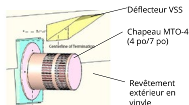
Figure 7.e Installation du déflecteur VSS.
