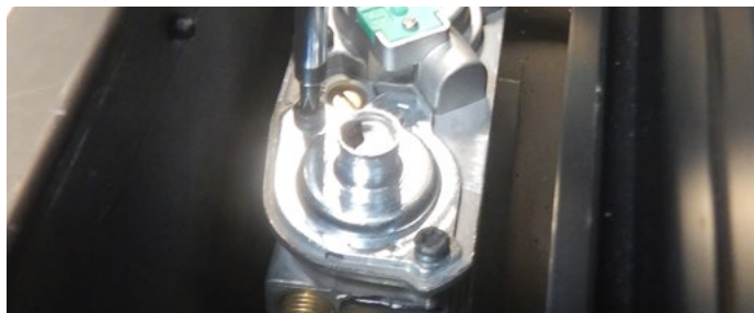
Figure 13.f Insérer l'obturateur pour gaz propane, puis remonter le brûleur
