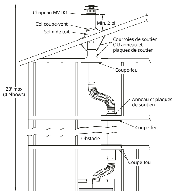
Figure 6.c Évent supérieur, monté sur le toit avec 2 déviations (1 déviation = deux angles de 90°).
