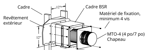
Figure 7.c Installation d'un chapeau MTO avec le cadre BSR.
