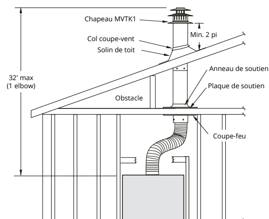
Figure 6.b Évent supérieur, monté sur le toit avec 1 déviation (1 déviation = deux angles de 90°).
