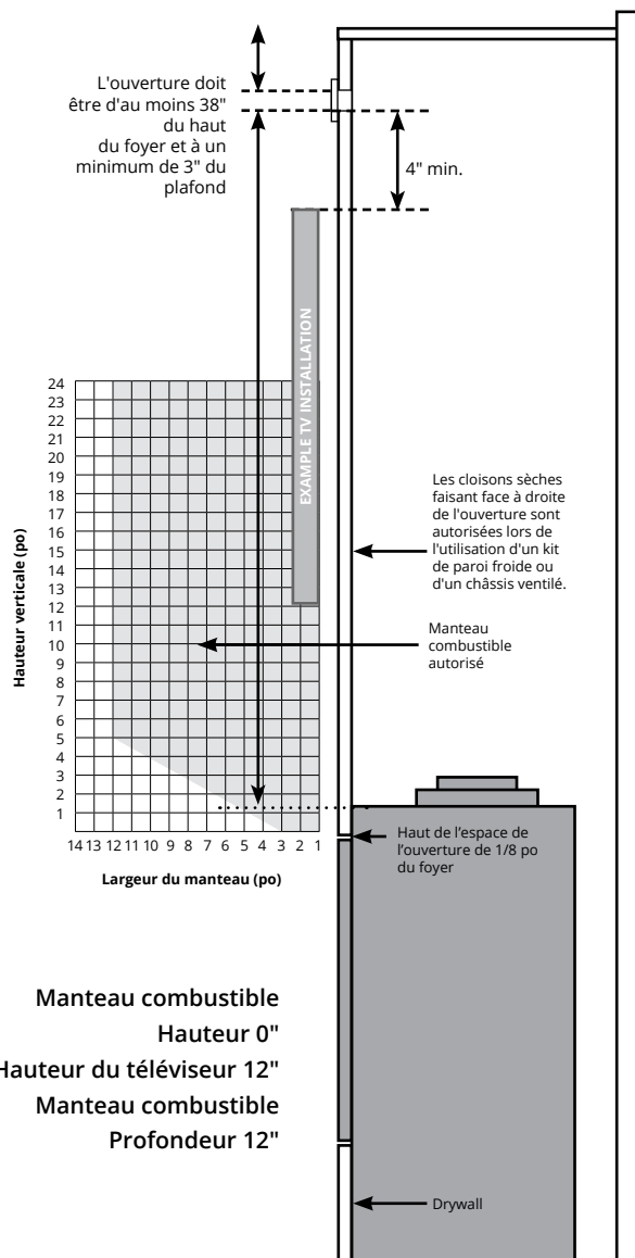
Figure 19.b Manteaux combustibles et revêtements. (N'est pas à l'échelle)
