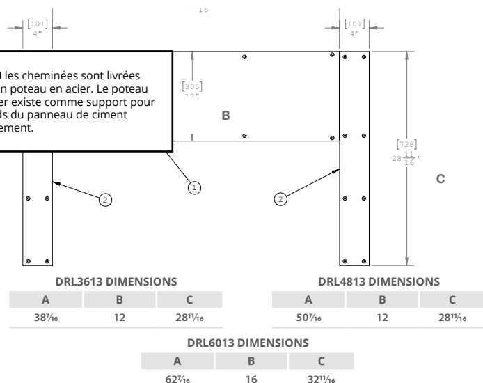
Figure 28. Dimensions du panneau de ciment non combustible fourni
