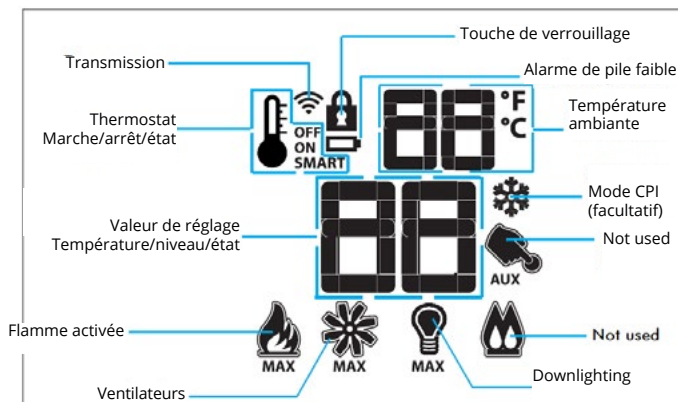
Figure 27.c Affichage à cristaux liquides de la télécommande
