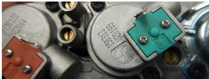
Figure 13.h Ajustez les ports de pression
