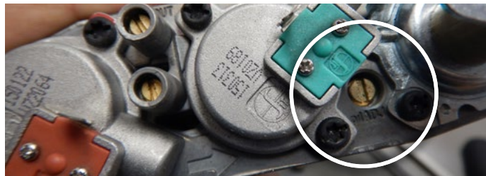
Figure 13.g Ajustez la taille de la veilleuse
