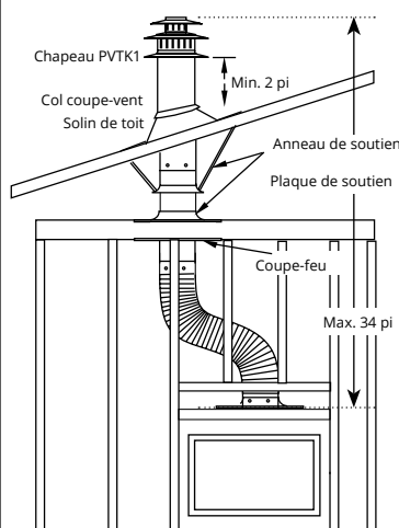
Figure 6.b Évent supérieur, monté sur le toit avec 1 déviation (1 déviation = deux angles de 90°).
