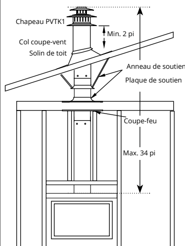
Figure 6. Évent supérieur, chapeau monté sur le toit sans déviation dans le parcours de ventilation.
