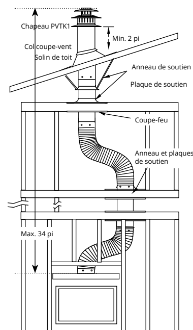
Figure 6.c Évent supérieur, monté sur le toit avec 2 déviations (1 déviation = deux angles de 90°).
