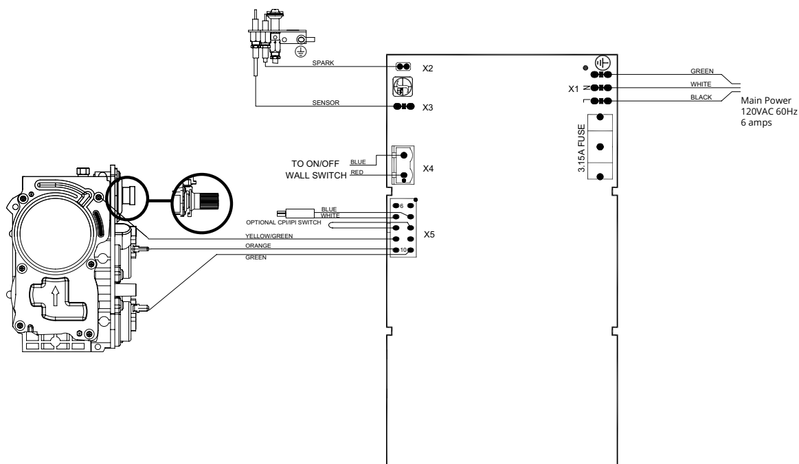
Figure 15. Schéma de câblage pour le modèle DRSQ38NI avec allumage électronique à TIA Profiflame
