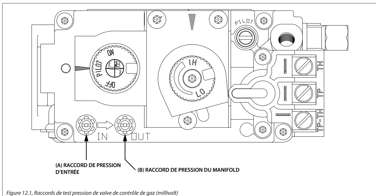
Figure 12.1, Raccords de test pression de valve de contrôle de gaz (millivolt)
