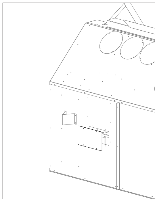
FIGURE 2.11 Retrait de la plaque-couvercle
