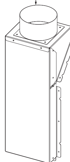
CHUTE D'AIR DU HTK (requis pour HTK-EXT)
