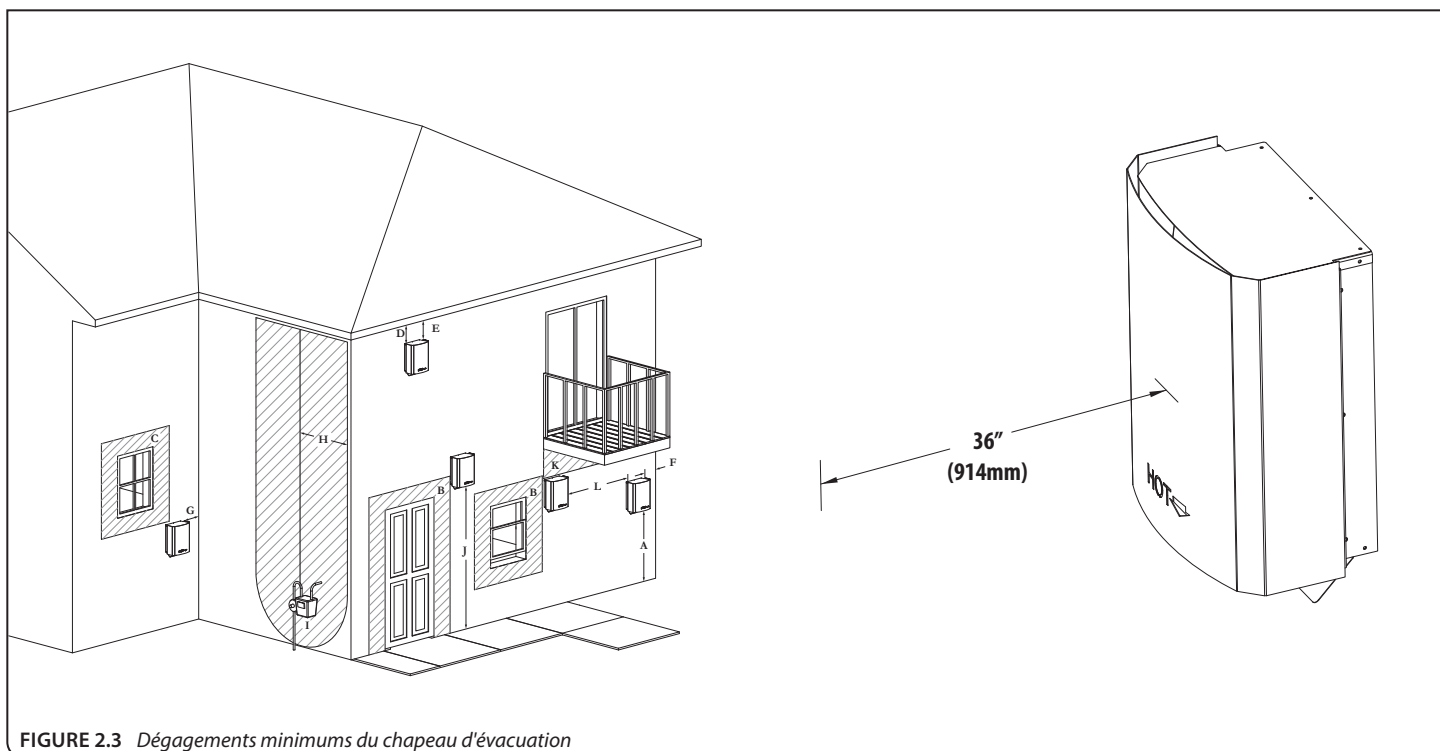
FIGURE 2.3 Dégagements minimums du chapeau d'évacuation
