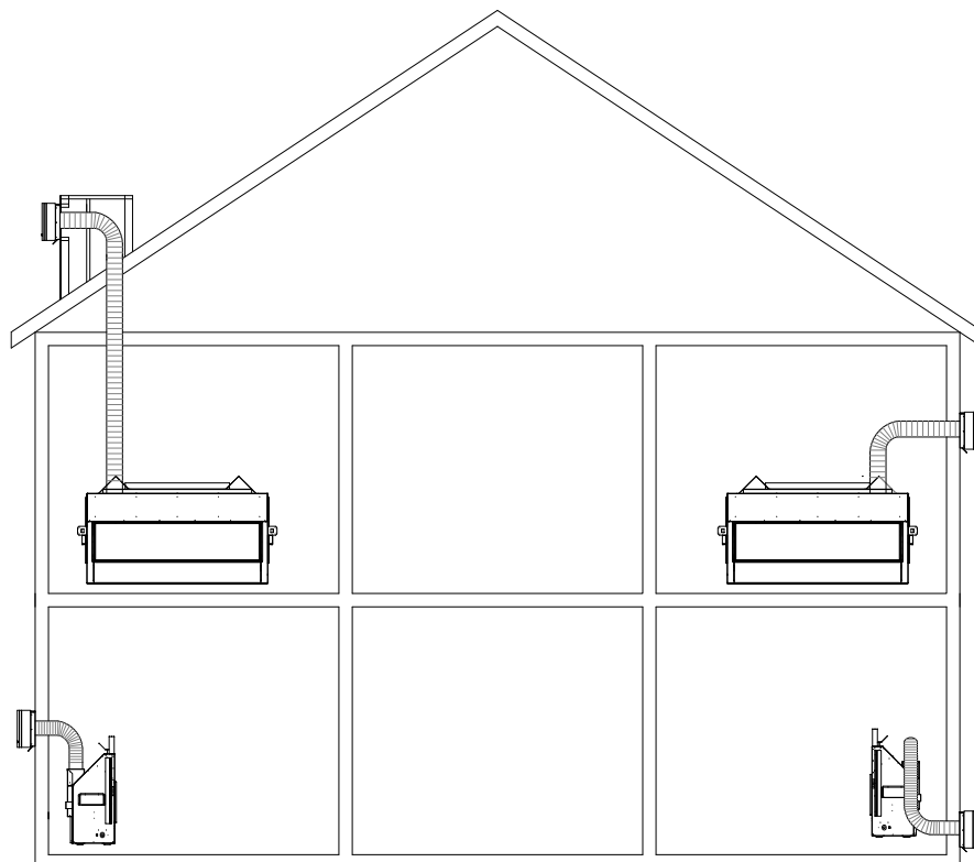
FIGURE 1.1 Emplacements possibles des conduits d'air et des chapeaux d'évacuation
