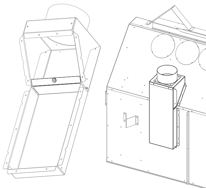
FIGURE 2.12 Installation de la chute d'air
