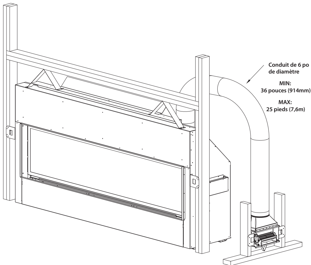
FIGURE 1.8 Dimensions du conduit
