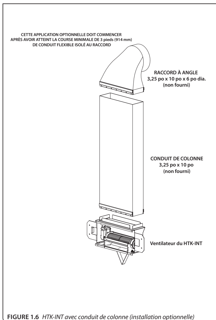
FIGURE 1.6 HTK-INT avec conduit de colonne (installation optionnelle)
