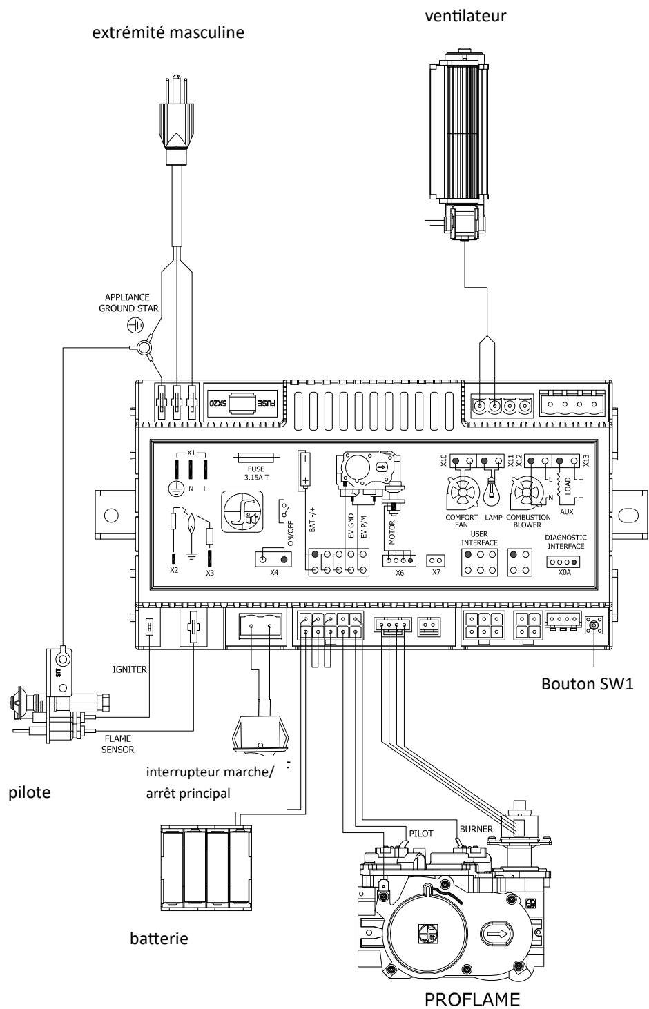
Figure 9.1 - Schéma électrique du SP-34-L
