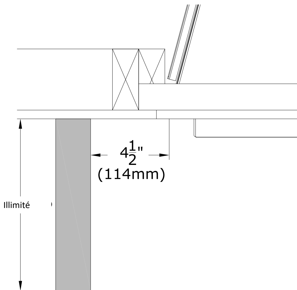
Figure 4.5 - Projection de paroi latérale combustible
