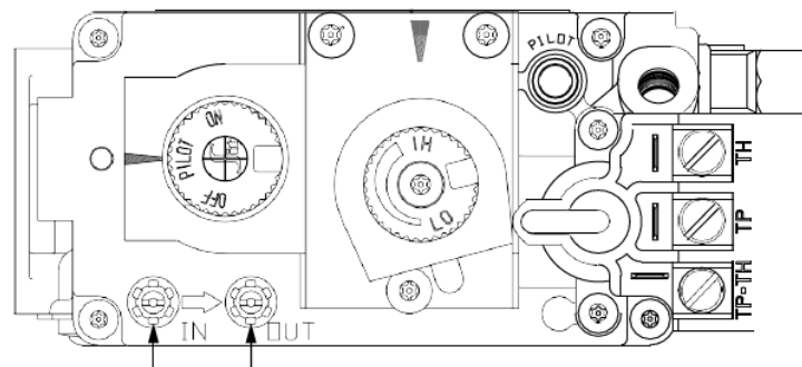
A) Robinet de pression d'entrée B) Prise de pression du collecteur
