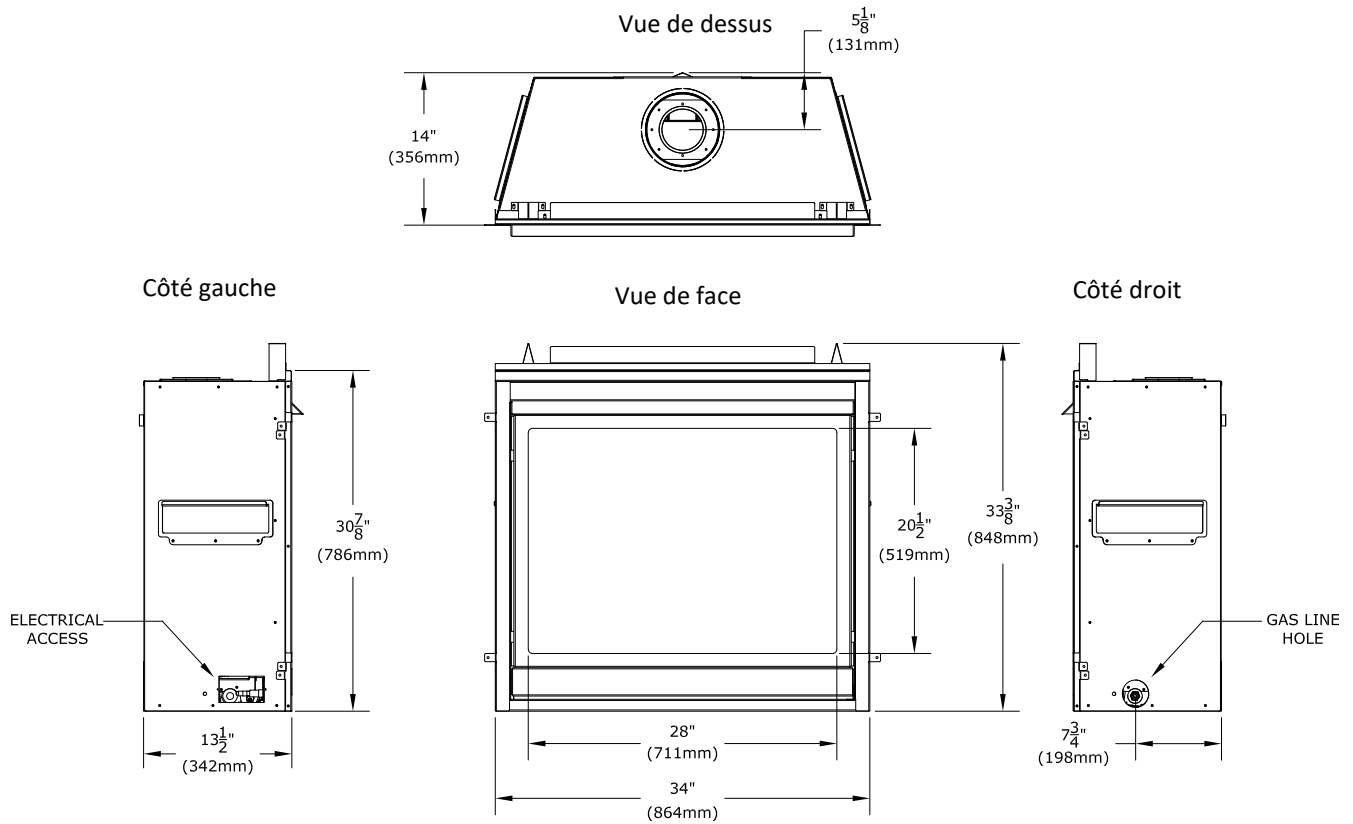
Figure 2.1 - Dimensions de l'appareil
