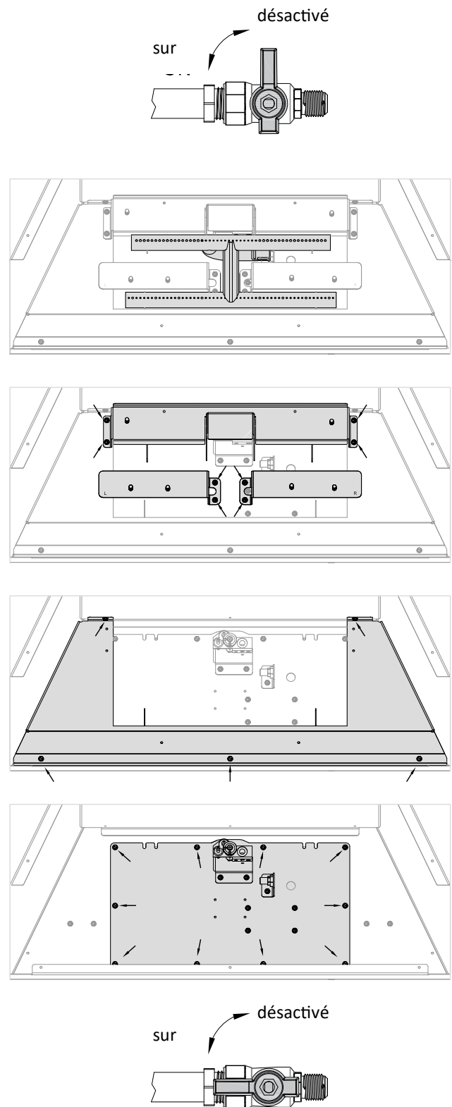
Figure 8.5 - Retrait du tableau de commande
