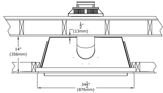
Installation horizontale typique
