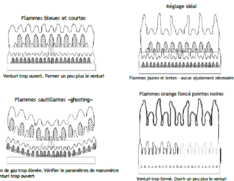
Figure 12.4 - Apparence et caractéristiques de la flamme
