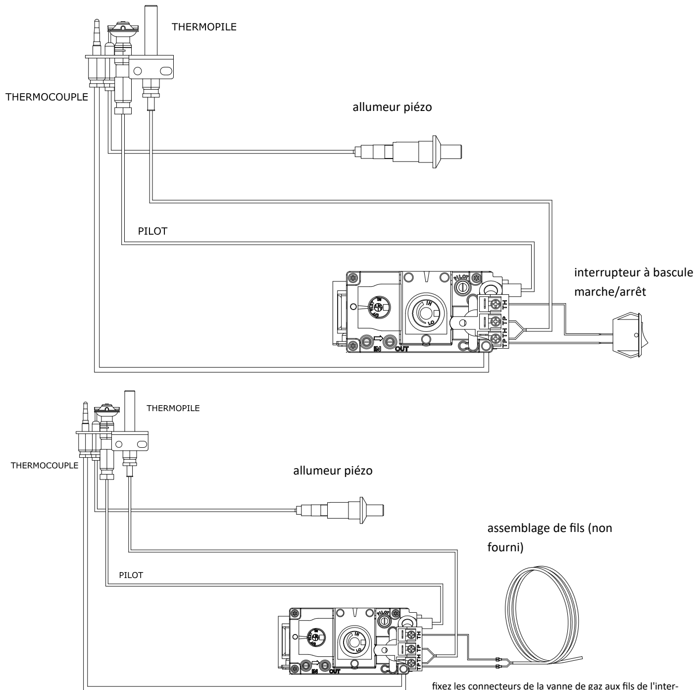
Figure 9.2 - Schéma électrique du SP-34-MV
