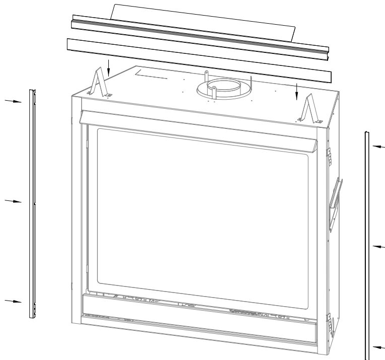
Figure 4.7 - Installation du kit de garniture extérieure
