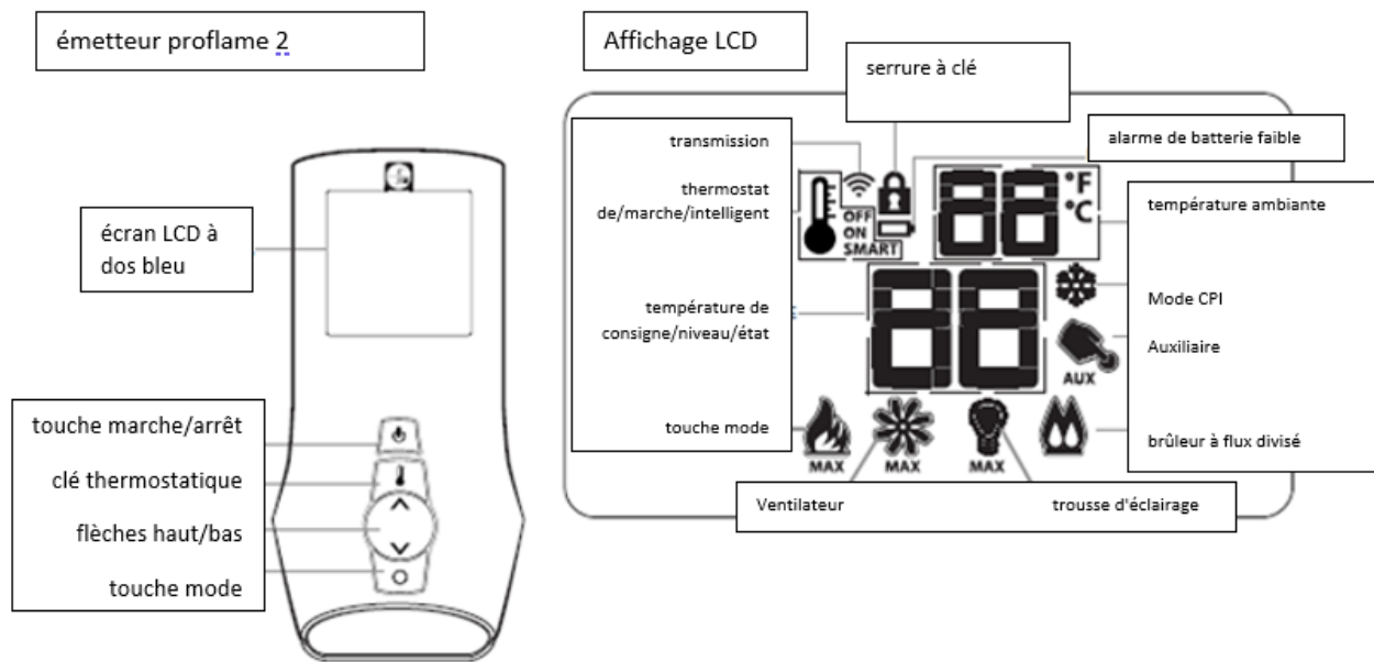
Figure 10.1 - Présentation de la télécommande
