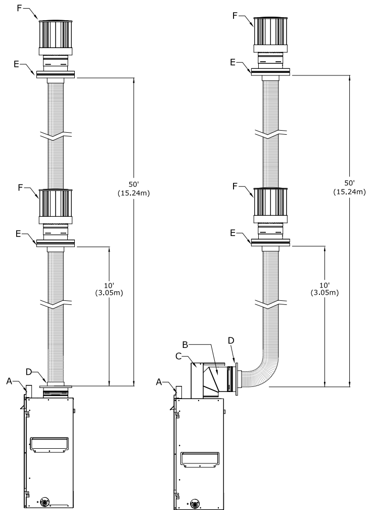
Figure 7.9 - Cheminée de classe A / Cheminée de maçonnerie
