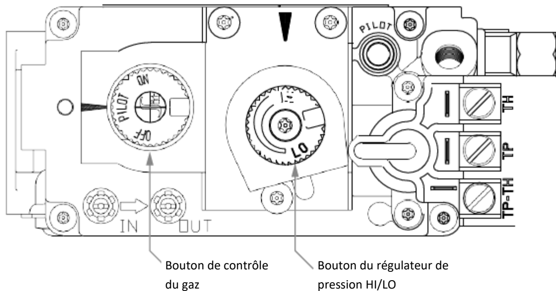
Figure 11.1 Vanne de régulation de gaz MT
