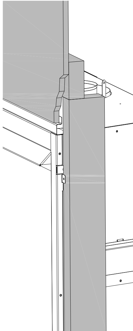
Figure 4.3 - Matériau de finition combustible
