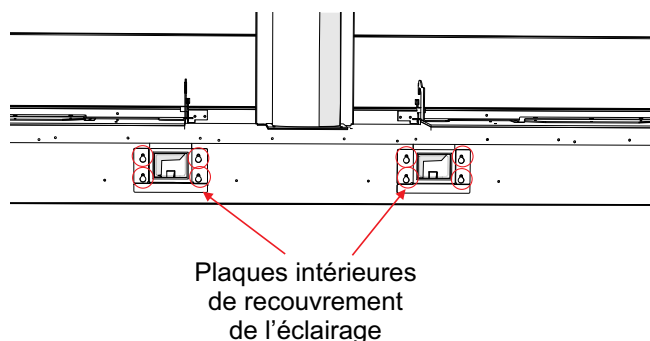
Plaques intérieures de recouvrement de l'éclairage depuis l'arrière de l'appareil (illustration en transparence)
