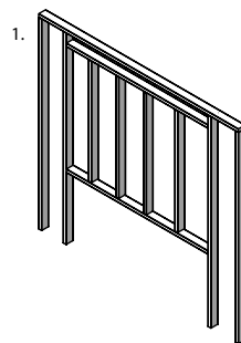
1. Ouverture de la structure d'encadrement pour l'évacuation (Voir page sur les dégagements de l'encadrement de l'évacuation)
