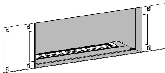
Installer les panneaux intérieurs
