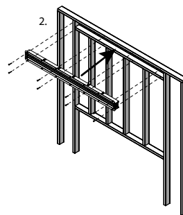
2. Visser l'évacuation du châssis à la structure
