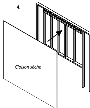
4. Construire la structure murale en utilisant un matériau de finition
