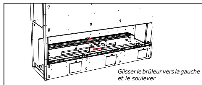
Emplacements des vis du brûleur
