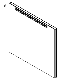
6. Découper une ouverture dans le matériau de finition, à l'intérieur de l'évacuation du châssis. Finaliser les rebords autour de l'ouverture.
