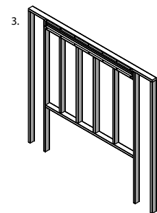
3. Utiliser au moins 4 jeux de vis pour garder l'évacuation à plat contre la structure d'encadrement
