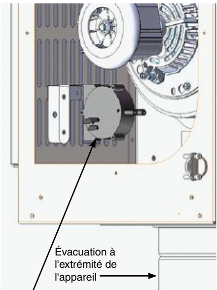
Orientation du pressostat si le système d'évacuation forcée en ligne est orienté verticalement (voir Schéma 1)
