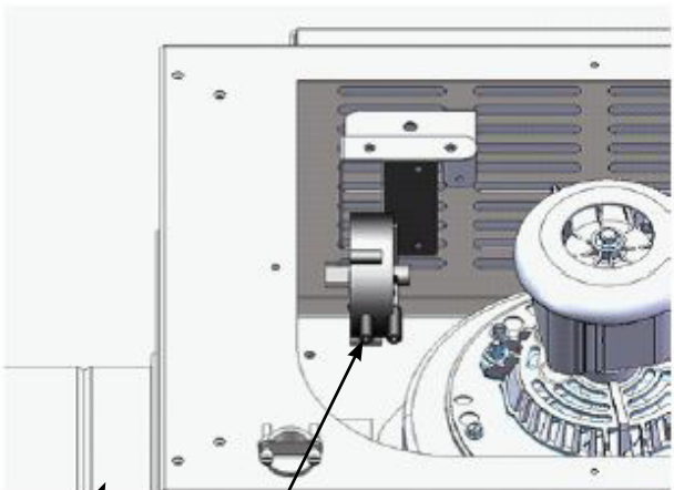
Orientation du pressostat si le système d'évacuation forcée en ligne est orienté verticalement (voir Schéma 1)
